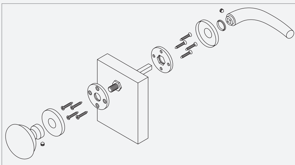
Pomolo fisso + maniglia girevole per porta blindata
