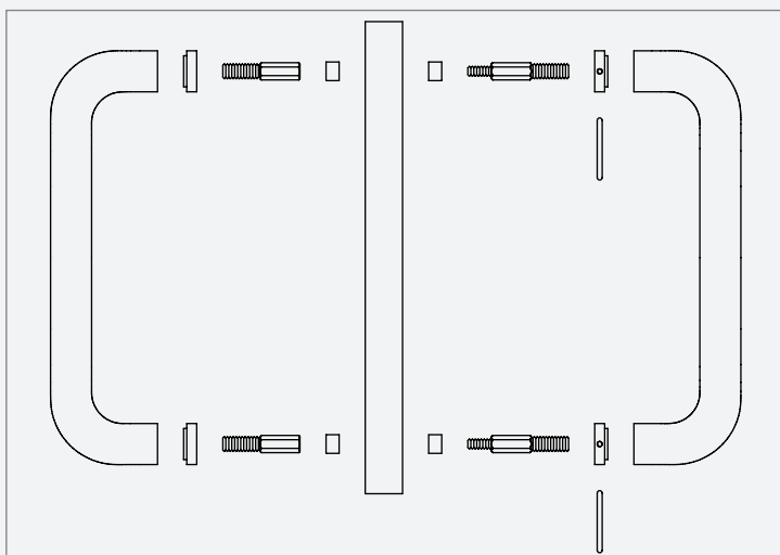
Coppia maniglione LIA per vetro, legno, alluminio
