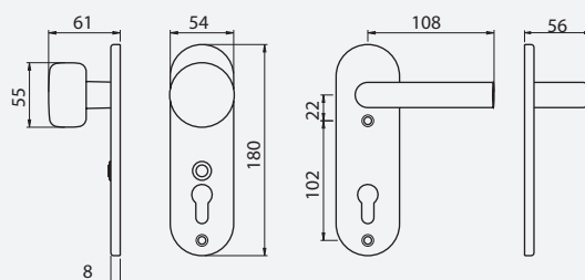
Placca tipo C.
