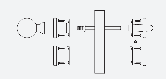
Guarnitura Hotel su rosetta/bocchetta
