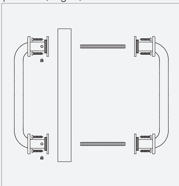
Coppia maniglioni con rosette per vetro, legno, alluminio
