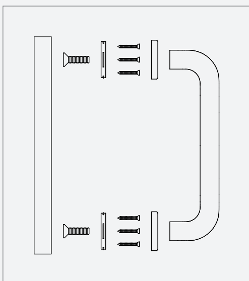
Maniglione LIA singolo con rosone
