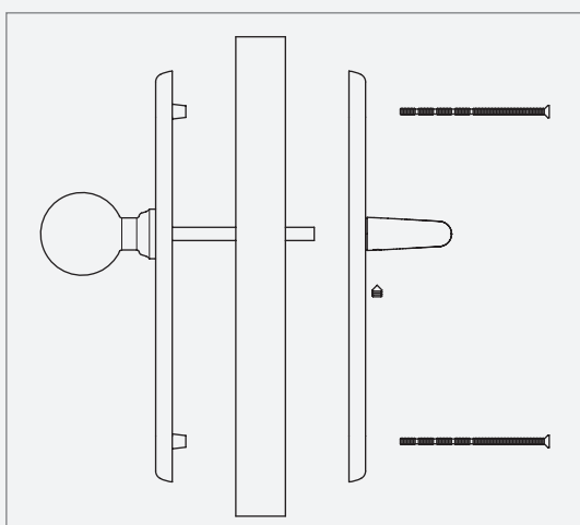
Guarnitura Hotel su placca con viti passanti
