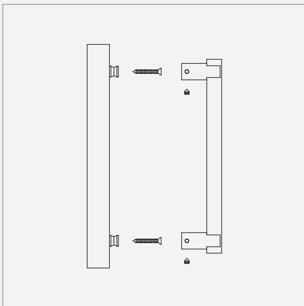
Maniglione senza rosette singolo
