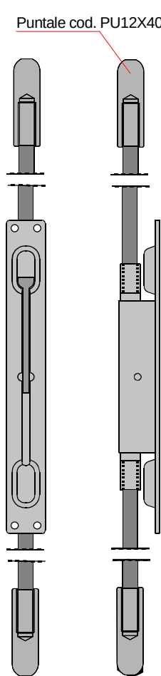
Catenaccio a leva a doppia azione Lever bolt double action
