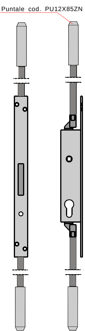
Serratura a doppio rinvio Lock, double action.
