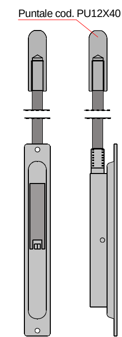
Catenaccio a leva a semplice azione Lever bolt simple action
