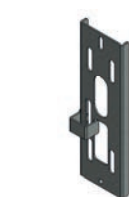
Piastra di protezione e di movimentazione aste. Handling and protection plate Plaque de protection et de mouvement des tiges
