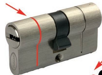
Sistema antirottura a taglio Anti-brake system made by cut Système anti-rupture avec coupure du corp du cylindre
